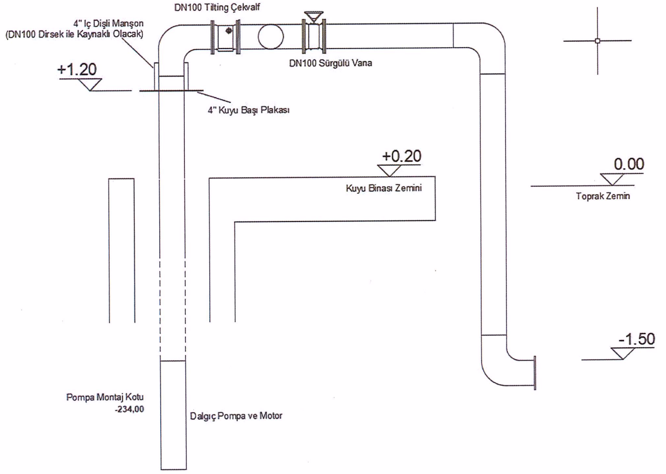
Ön Görünüş
