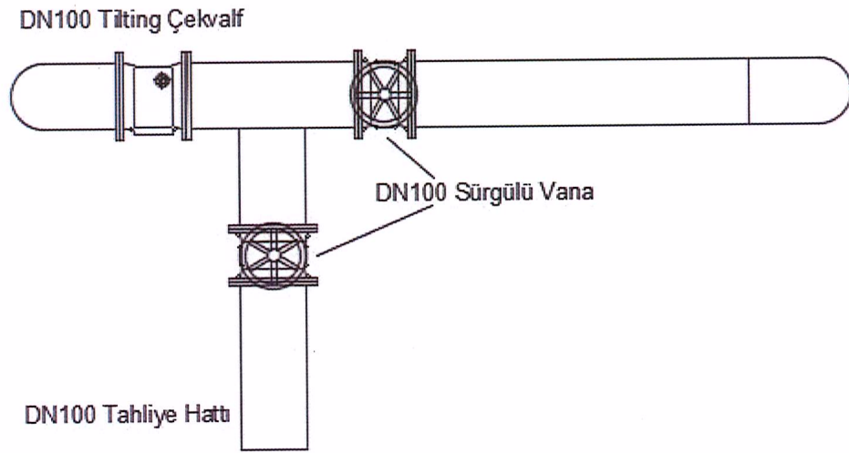
Üst Görünüş
