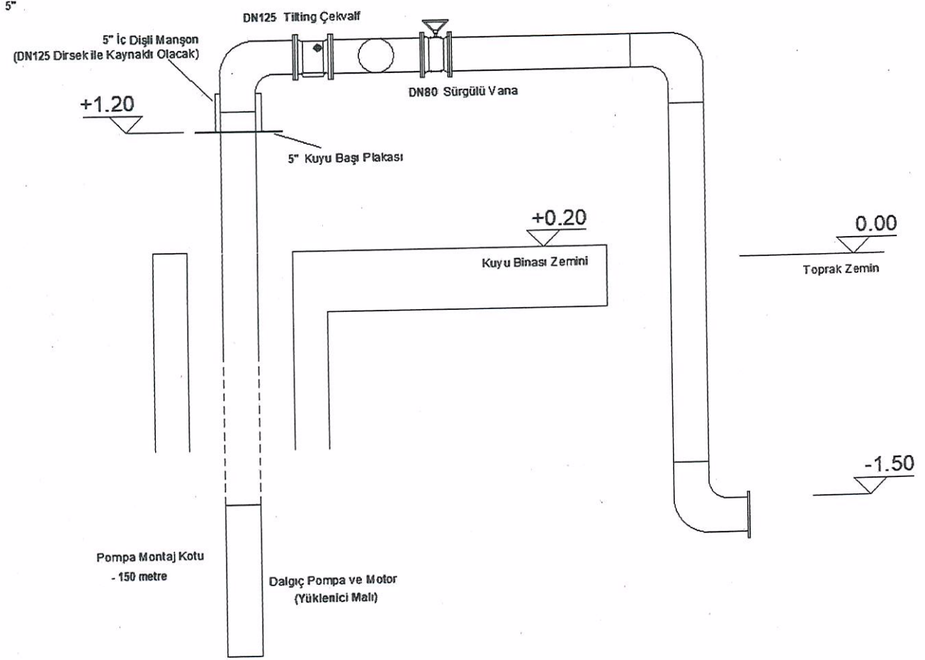
Ön Görünüş
