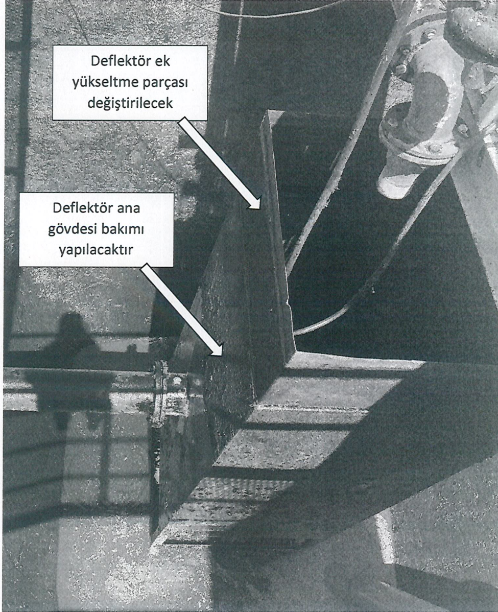
Görsel 4 : Çöktürme Havuzu, Deflektör ve yükseltme parçası.
