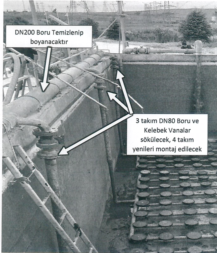
Görsel 1: Havalandırma Havuzu, Çelik hava boruları ve vanalar
