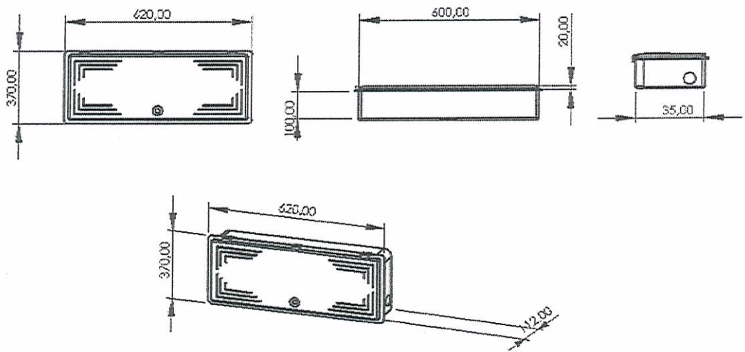
Şekil-2: Plastik Vana Sayaç Kutusu Montaj Ölçüleri
