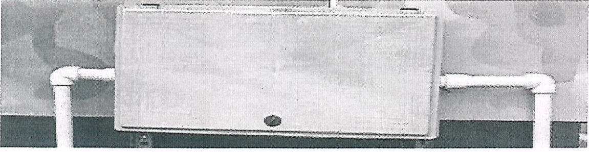
Şekil-4: Plastik Vana Sayaç Kutusu Montaj Cephe Görünümü(Kapalı)
