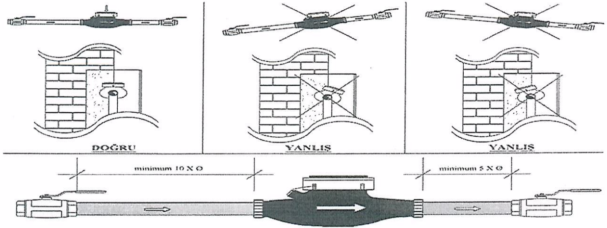
Şekil-1: Sayaç Montaj Eksen Çizimi
