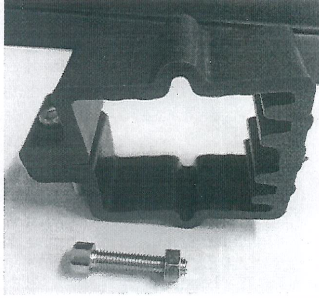
Temsili Fotoğraf 3. Panel çit kelepçesi (vida ve somun dahil)
