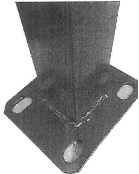
Temsili Fotoğraf 2. Kare profil panel çit direği (bağlantı plakalı, üst plastik kapaklı)
