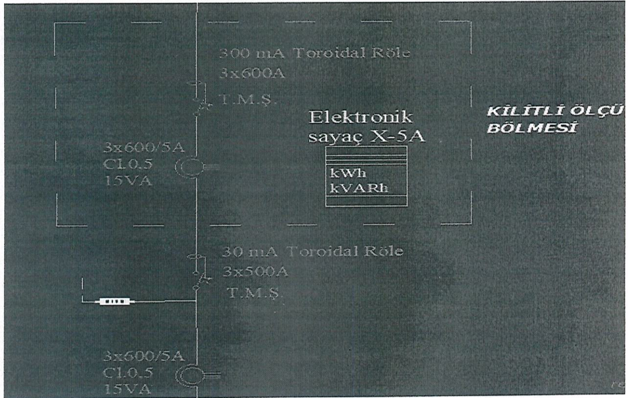
Çizim 2. Elektrik Projesinden Detay
